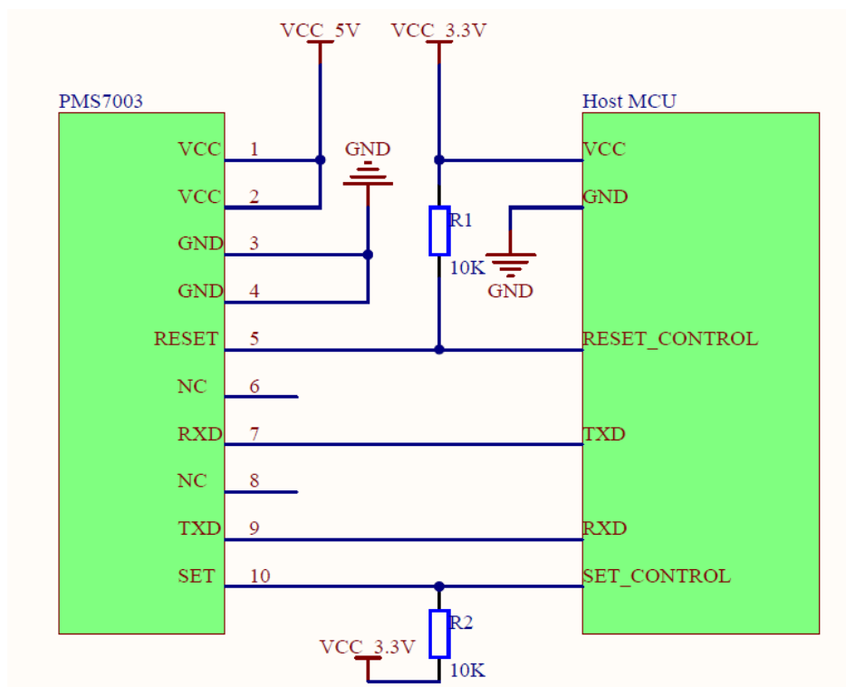
图 3 典型电路连接图
